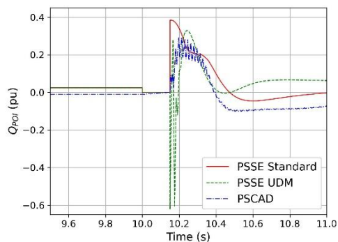
(d) Reactive power at the POI
